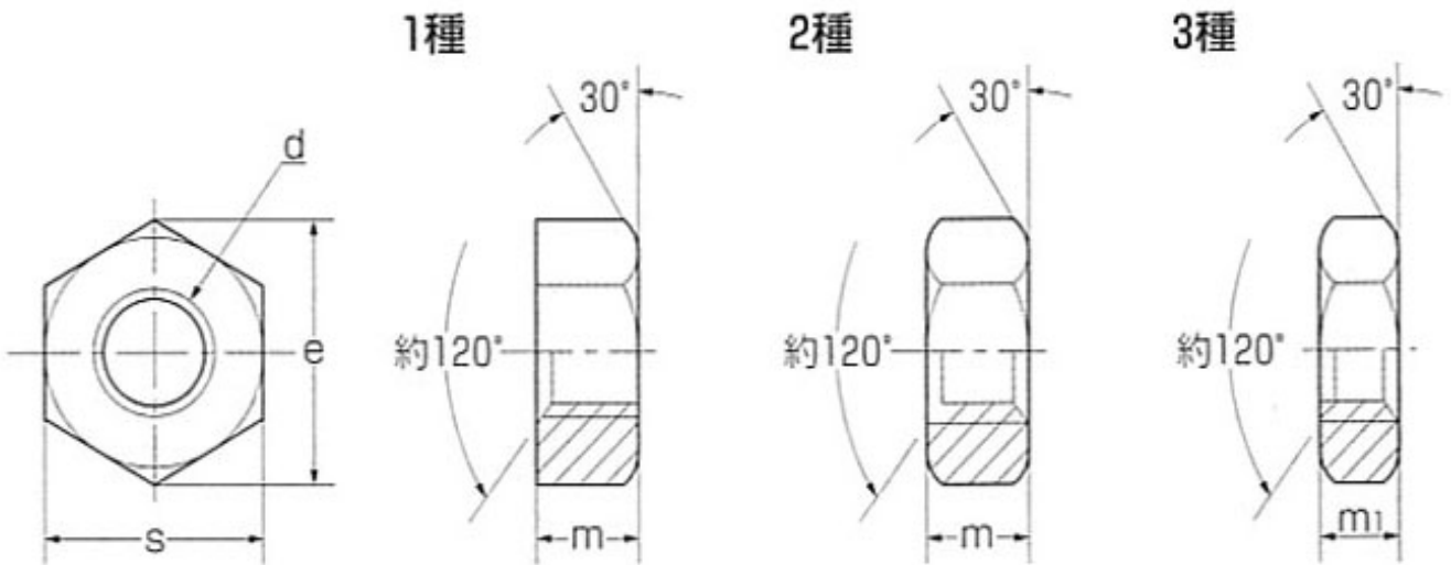
■六角ナットMねじ寸法表 JIS B 1181-1993
